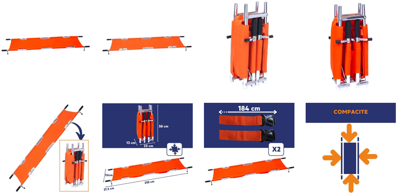
Brancard pliable 10-8 pliant en 8 Brancard pliable 10-8 pliant en 8 Brancard pliable 10-8 pliant en 8 Brancard pliable 10-8 pliant en 8
